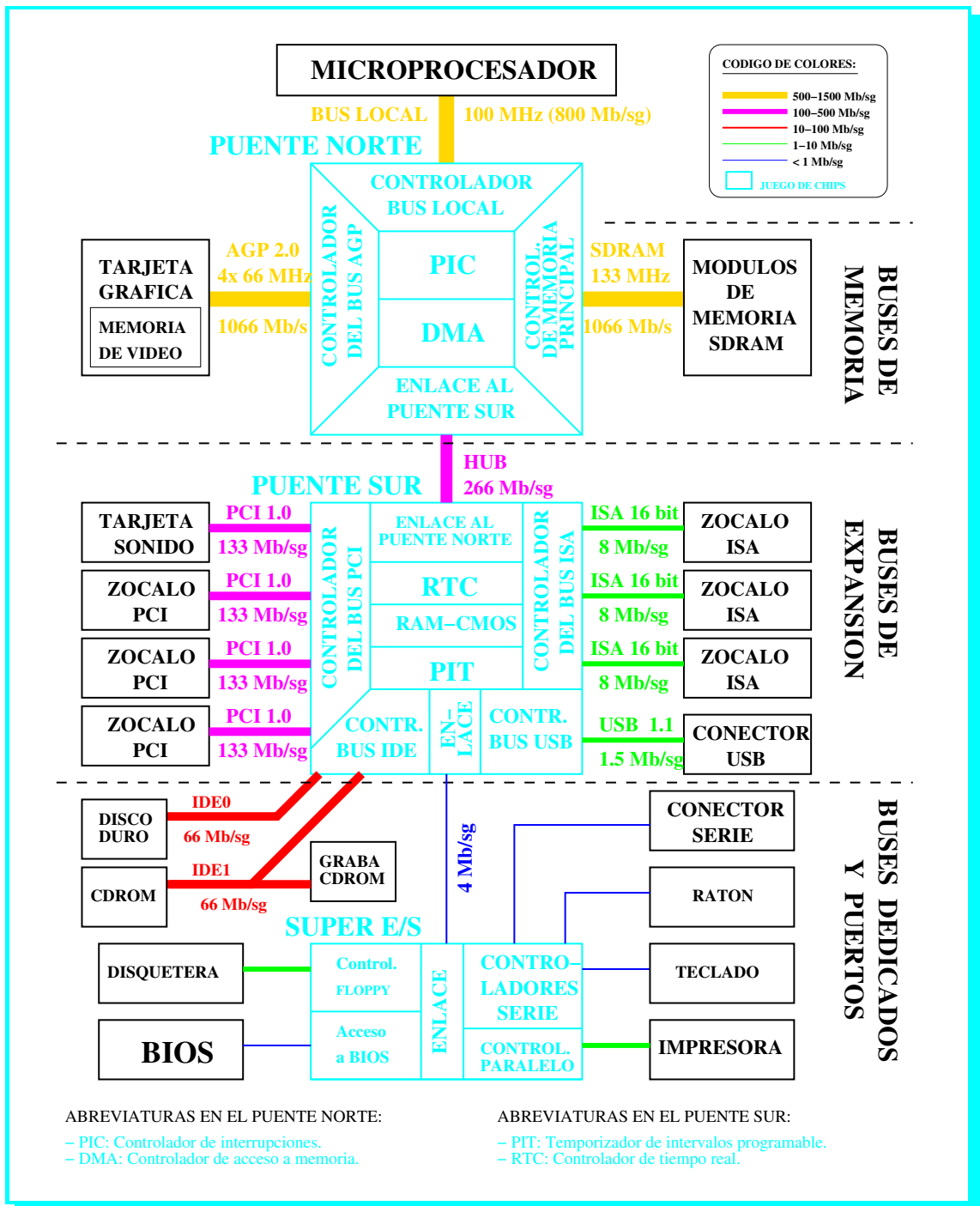
FIGURA 18.8: El patrón más común para la arquitectura del juego de chips en el contexto de la sexta generación.
