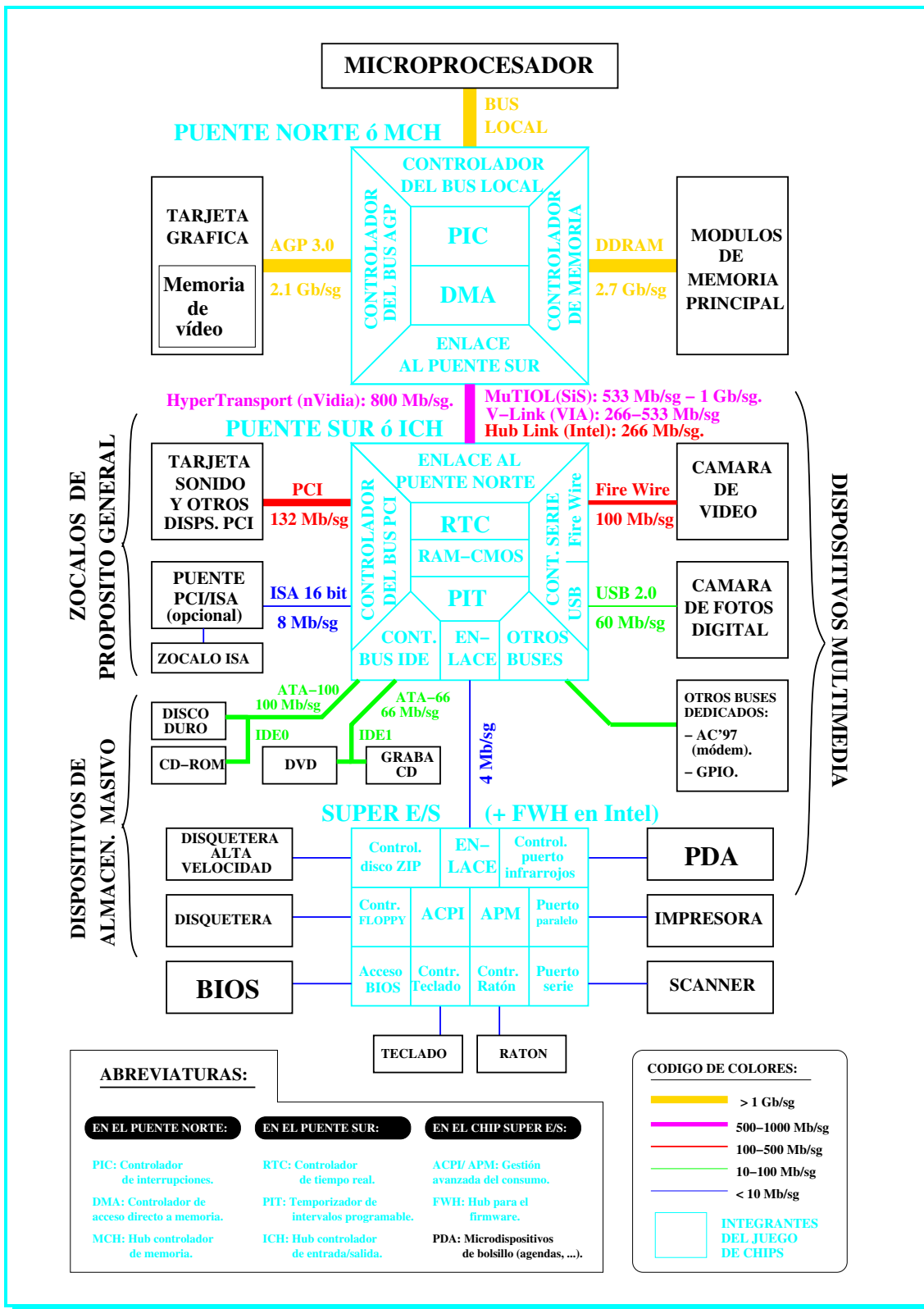
FIGURA 18.11: El patrón más común para la arquitectura del juego de chips en el contexto de la séptima generación.
